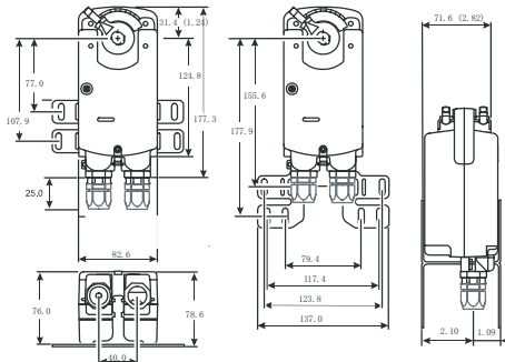
尺寸 (mm)
