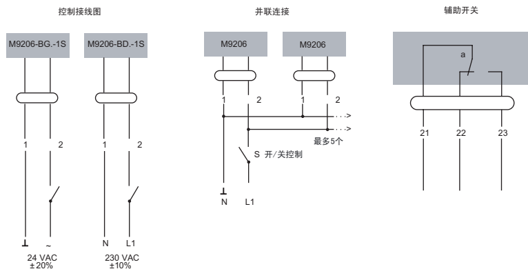
接线图
